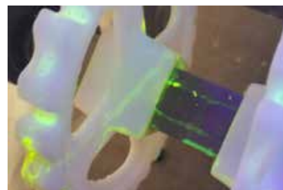
Lo sporco è stato additivato con una tintura fluorescente. Dopo la pulizia, è stata utilizzata una luce ultravioletta per individuare lo sporco residuo.
